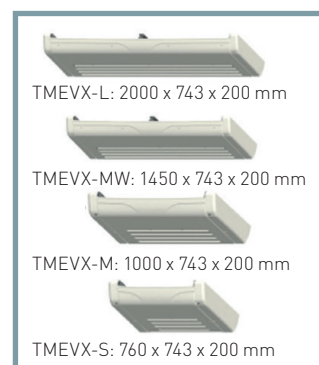
Evaporator
